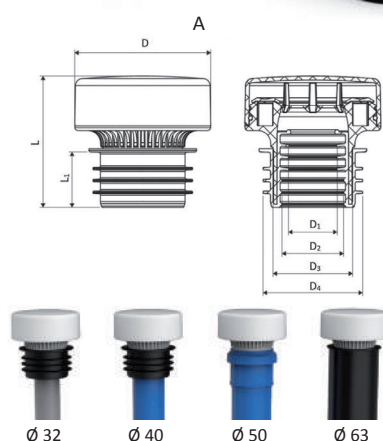
Válvula de admisión de aire AIRVAL
