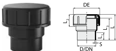
Tapón de cierre completo
