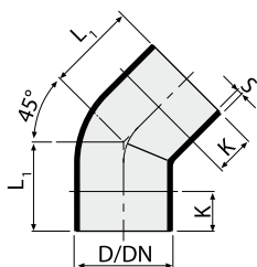
Codo 45°
