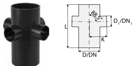
Derivación 88° 30' 4 salidas
