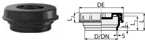
Tapón de cierre completo
