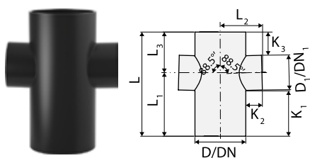
Derivación doble 88° 30'
