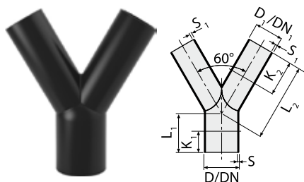
Derivación doble en Y 60°
