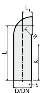
Curva rasa 90°
