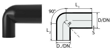
Curva reducida 90° prolongada
