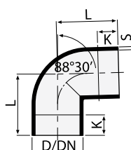
Curva 88° 30'
