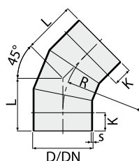
Codo 45° de radio largo
