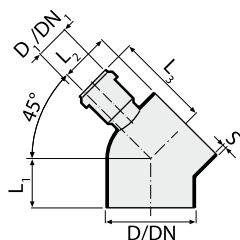
Curva 45° con derivación
