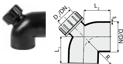
Curva 88°30' con inspección Ø63
