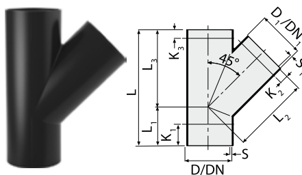
Derivación 45°
