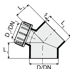
Curva 45° con inspección Ø63
