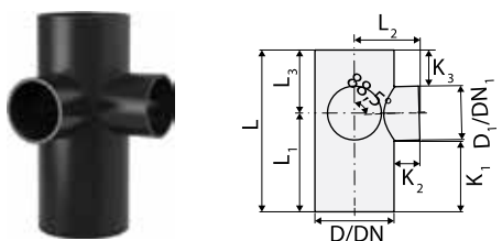
Derivación en ángulo 88°
